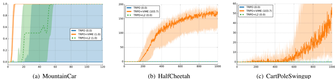
图 7.1 VIME 实验中的学习曲线。图片改编自文献 (Houthooft et al., 2016) (见彩插)
